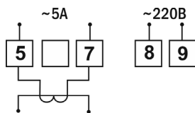
Рис. 3 – Подключение Omix P94 через трансформатор тока
