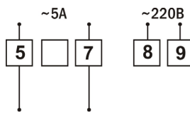
Рис. 4 – Прямое подключение Omix P94
