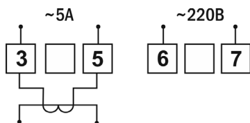
Рис. 5 – Подключение Omix P99 через трансформатор тока
