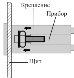
Рис. 2 – Установка прибора
