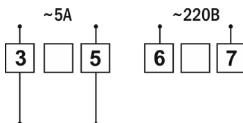
Рис. 6 – Прямое подключение Omix P99
